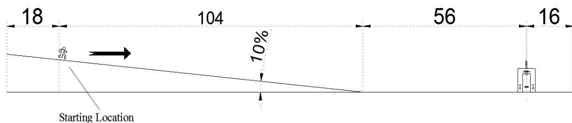
Figure 2 . Side view of the Träderskolevägen tunnel.
