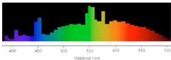
Figur 4. Spektrum från lysrörlågenergilampa innehållande kvicksilver.
