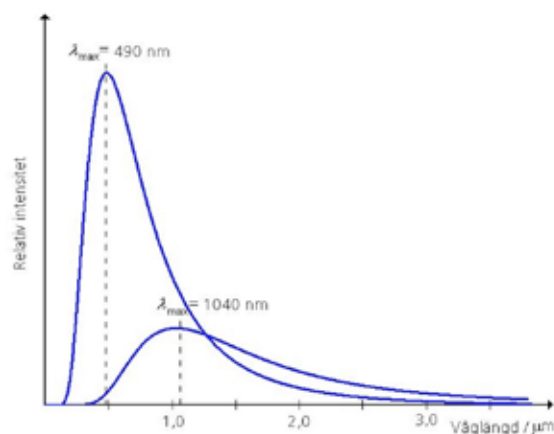
Figur 2. Spektrumets utseende för solen max= 490 nm (respektive för en glödlampa max=1040nm)
