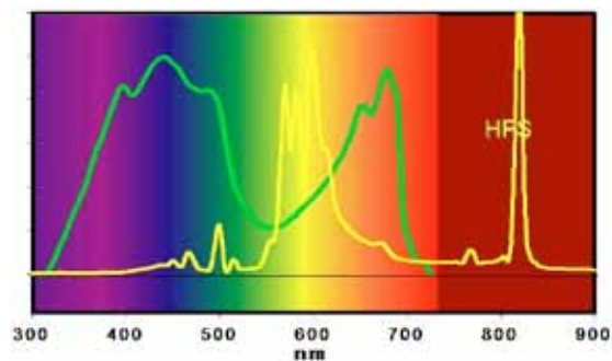
Figur 6. Fotosyntesens nytta av olika våglängder och spektralfördelningen för en HPS-lampa.
