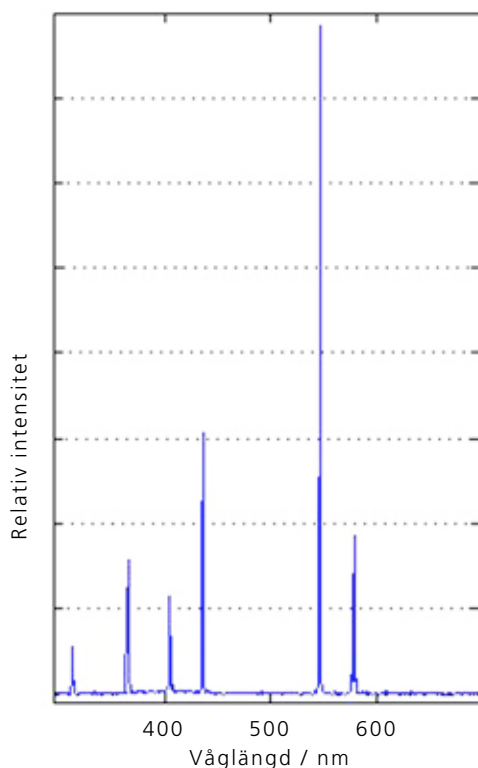
Figur 3. Kvicksilverspektrum.
