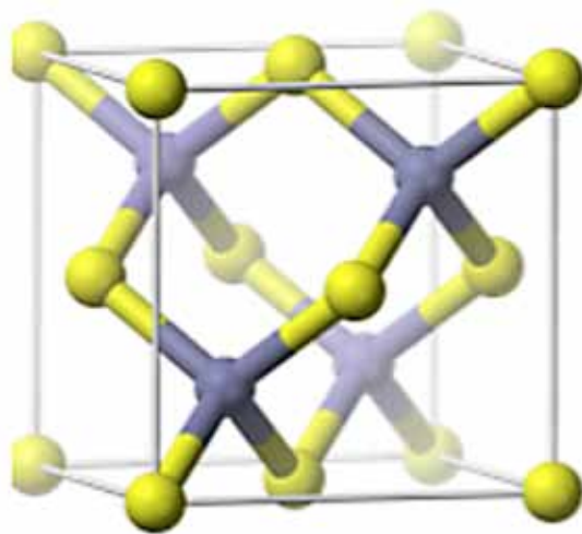
Figur 24. Zinkblendestruktur (för t ex GaAs)
