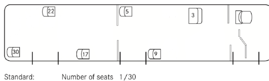
Citaro LE, 3 doors (C 628.504-13, C 628.506-13*)
