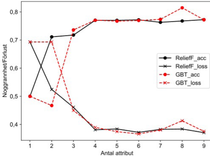
Figur 6. Noggrannhet och förlust för ANN-modellen när fler attribut läggs till i den ordning som ReliefF (svart, heldragen linje) och GBT-PI (röd, streckad linje) indikerar. Noggrannhet (acc), vilket anger hur bra ANN-modellen är på att förutsäga vilka ledningar som har haft läckor, visas som linje med punkter. Förlust (loss), vilket är ett mått på hur långt ifrån yttervärdena noll och ett modellen är i sin klassificering, visas som linje med kryss.
