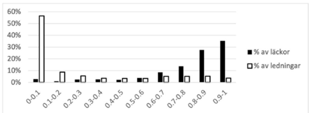
Figur 3. Procentandel ledningar i varje grupp av prediktionsvärde för SVOA (vita staplar) och procentandel läckor inom varje grupp (svarta staplar) som uppstått efter att ANN-modellen körts.
