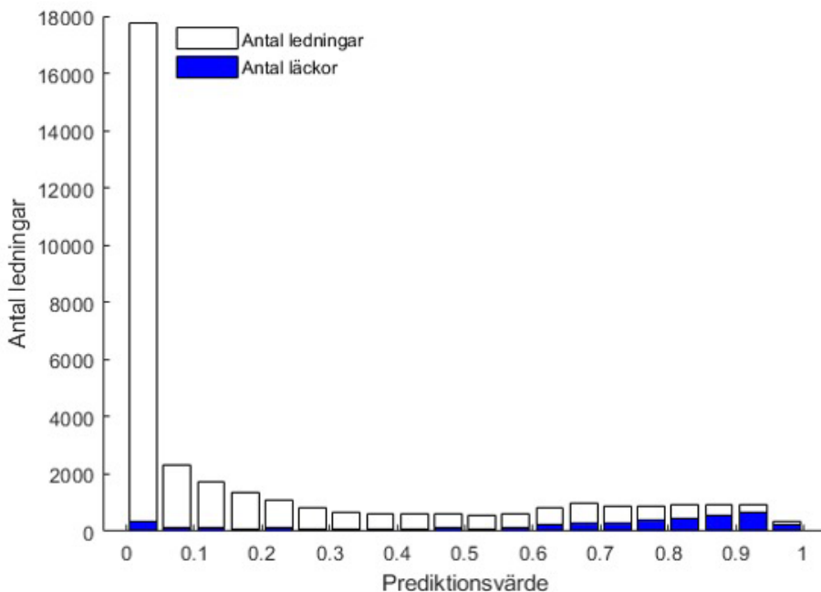
Figur 1. Antal ledningar i varje grupp av prediktionsvärde för SVOA:s data. I blått visas antalet ledningar med registrerade läckor, vilket används som indata för att träna ANN-modellen. 26,5 % av alla läckor ses på ledningar som har ett prediktionsvärde under 0,5.
