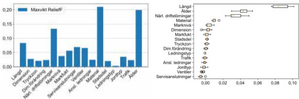
Figur 5. Utvärdering av ledningsattributens vikt för SVOA:s ledningsnät utifrån två olika metoder. Vänster: Maxvikt för attributen utifrån ReliefF. Höger: Attributens vikt utifrån GBT-PI. I båda fallen indikerar högre värde att attributet är av större vikt.
