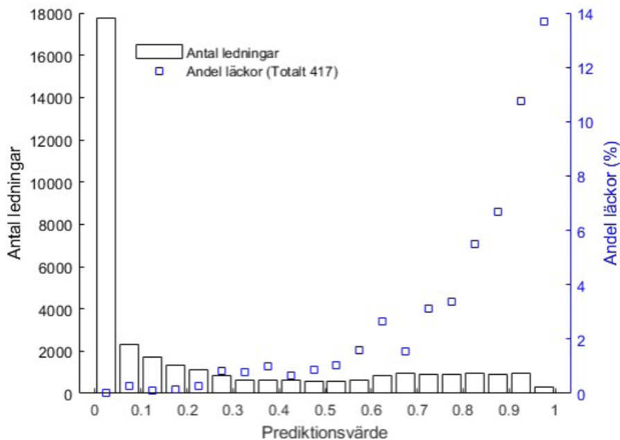
Figur 2. Antal ledningar i varje grupp av prediktionsvärde för SVOA (som staplar, vänstra axeln) och andel läckor inom varje grupp (%) som uppstått efter att ANN-modellen körts (som punkter i blått, högra axeln). Sammanlagt så har 417 läckor uppstått under utvärderingsperioden januari 2019 till maj 2021.
