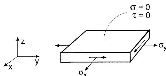
Figur 37: Plant spänningstillstånd på en fri yta.
