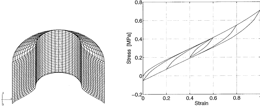
Figur 33: Amplitudberoende dynamisk styvhet. FE-analys av cylindrisk komponent i axiell cyklisk skjuvbelastning.
