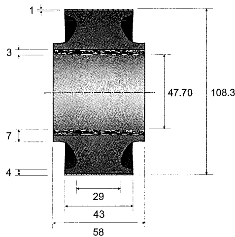
Figur 1: Snitt av bussningen. Textil- och metallarmering i ytter- resp. innerkant.
