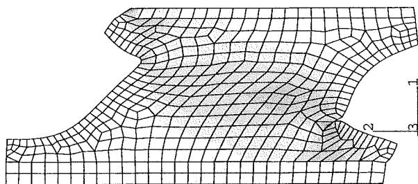
Figur 6: Töjningsenergiens fördelning.
