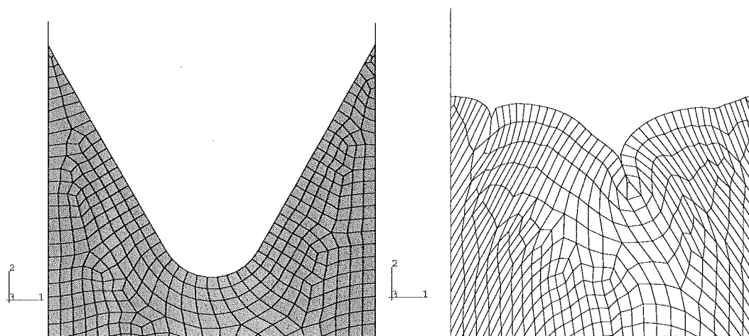
Figur 14: Symmetriskt förslag nummer 1. Till vänster innan kompression och till höger vid full kompression \Delta r = 3.28mm .
