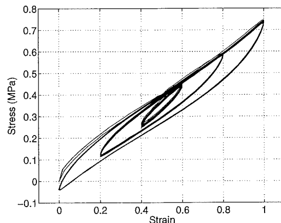
Figur 24: Kvasi-statiskt test i skjuvning med harmonisk belastning vid 0.05\text{Hz} med ökande amplitud.
