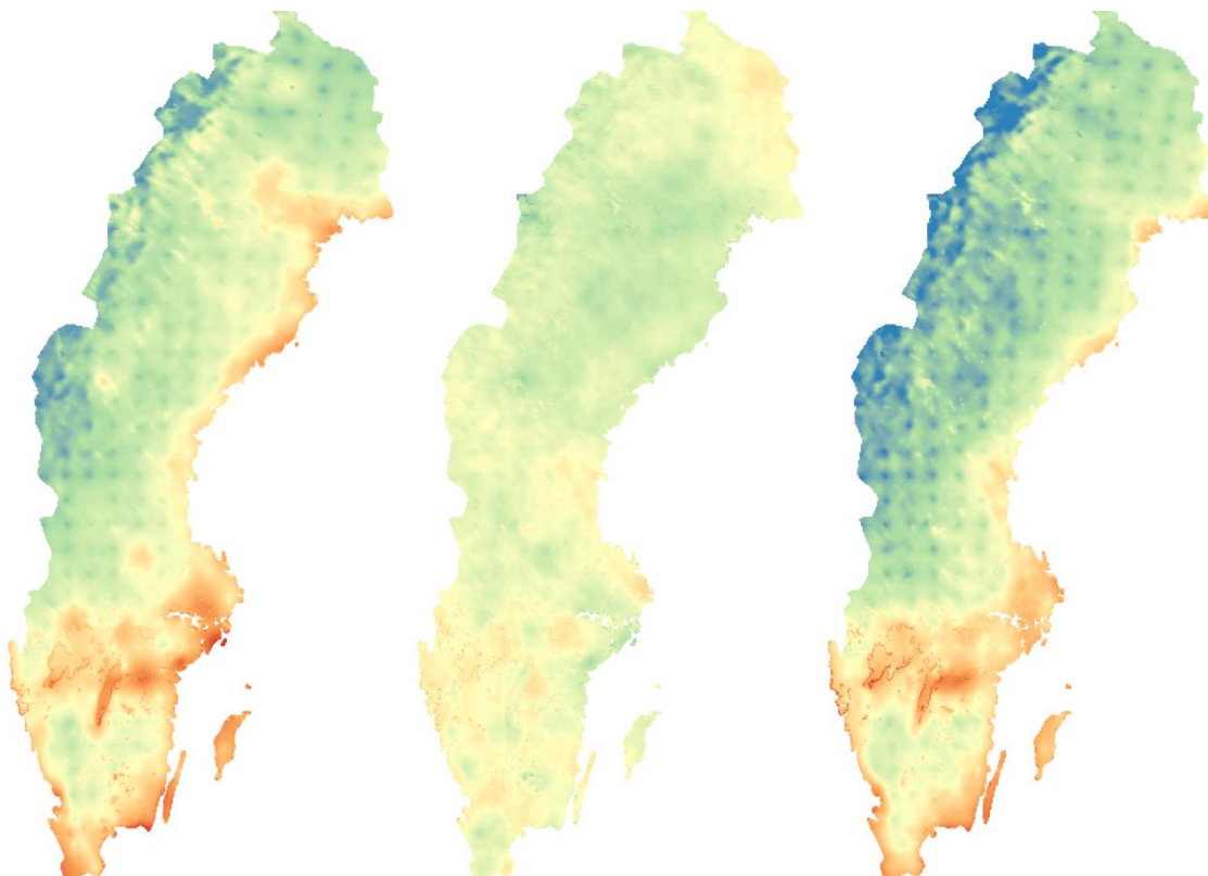
Figur 2. Antal soltimmar i Sverige under ett år som medelvärde för perioden 2017-2022 (vänster), under 2022 (höger) och som ett mått på hur mycket 2022 skilde sig från ett normalår (mitten). Blått motsvarar färre soltimmar, rött fler. Max för 2022 är 2020 soltimmar (Tun, Västergötland), minimum är 811 (Vuoggatjålme, Pite lappmark). Samma skala används för 2022 och medelvärdet 2017-2021. Kartan som visar 2022 års avvikelser (mittenkartan) har som mest 346 soltimmar mer än normalt (Äspered, Ulricehamn) och som minst 518 soltimmar färre än normalt (Överuman, Ume lappmark). Data kommer från SMHI:s databas STRÅNG (2021).
