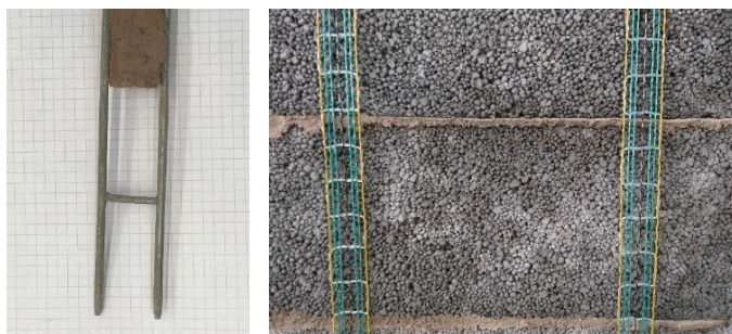
Bild 2.1 Förstärkningsmaterial: avslitet bistål (vänster); vajerarmering (höger).
