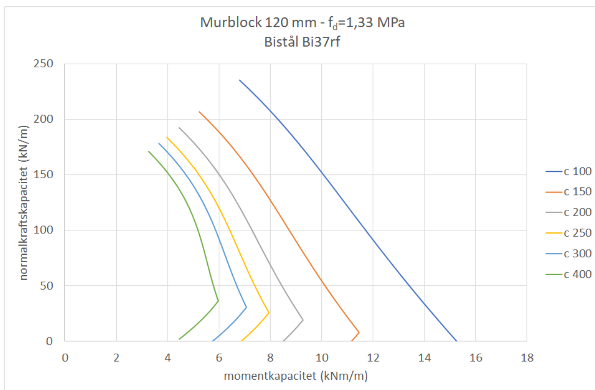
Diagram A1.6 Traditionellt murat Leca murblock 12 cm, hållfasthetsklass 3 MPa; ytförstärkning av rostfritt bistål av typen Bi37rf.
