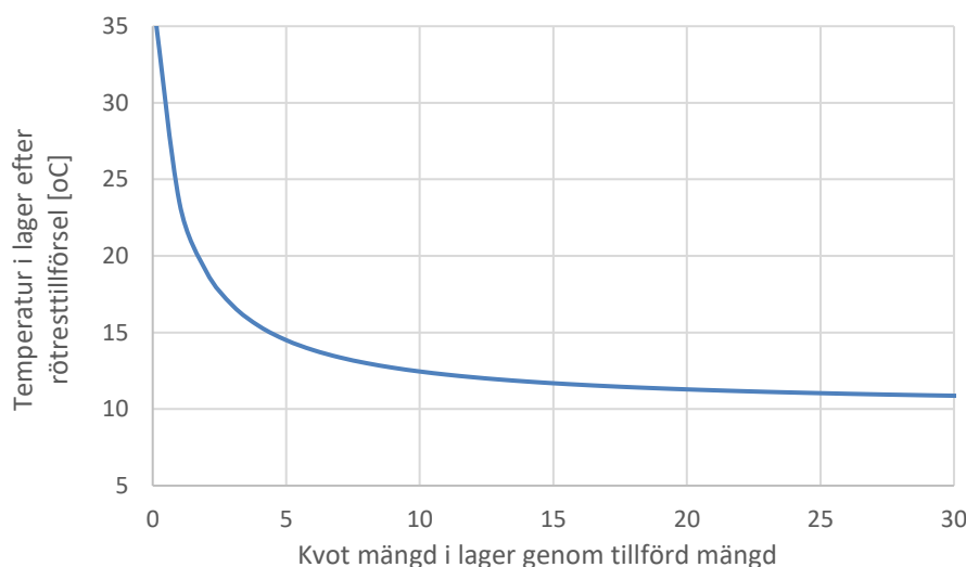
Figur 3: Lagertemperaturen vid olika tillförsel av varm (37 °C) rötrestart i ett rötrestartlager vid 10 °C
