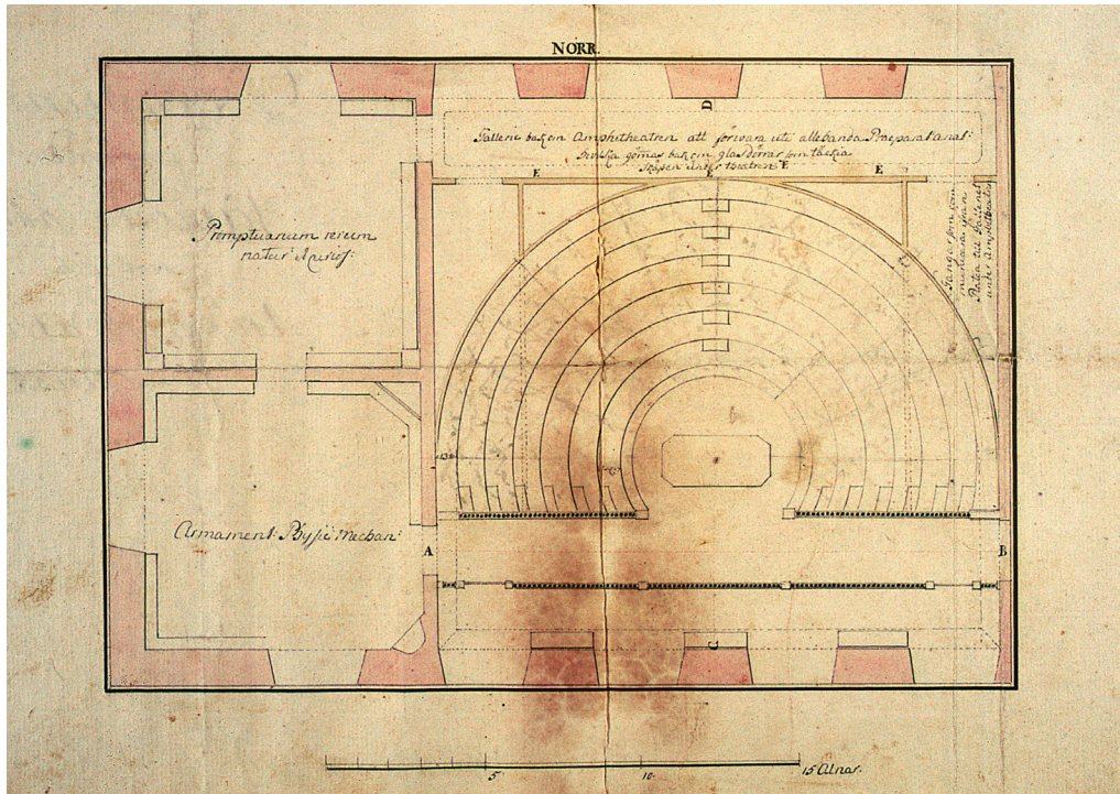
Carl Hårlemans ritningar från 1733 över den anatomiska teatern på andra våningen i Lundagårdshuset. Bakom den marmorerade amfiteatern, i norr, förvarades de anatomiska preparaten; till vänster två rum med instrumentsamlingen i fysik och mekanik samt naturalie- och kuriosa-samlingen. Foto: Lunds universitetsarkiv/Alvin.
