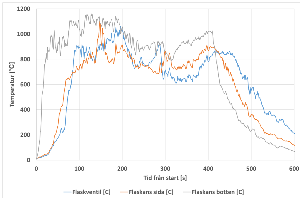
Figur 8: Temperurmätningar på flaskan.
