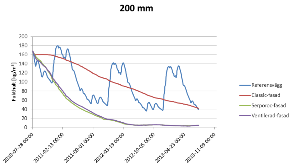
FIG 7.8. Beräknad fukthalt med standarddata på djupet 200 mm i de olika väggarna.
