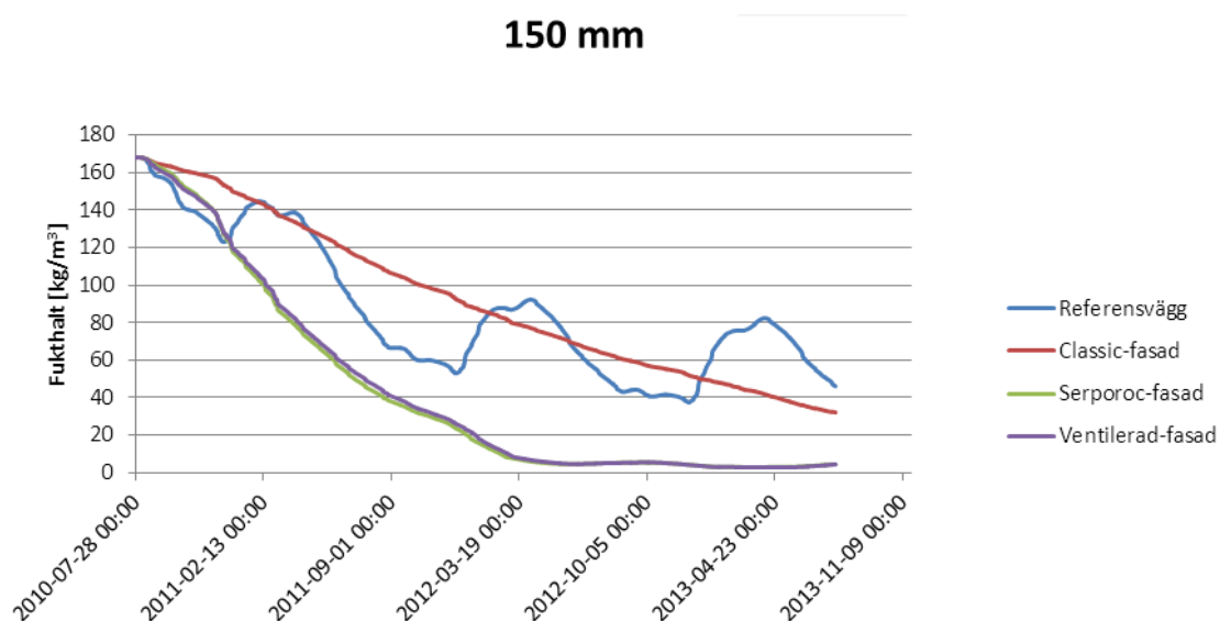
FIG 7.7. Beräknad fukthalt med standarddata på djupet 150 mm i de olika väggarna.
