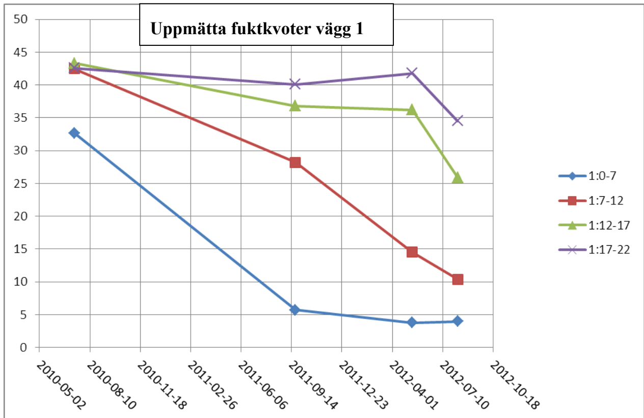
FIG 6.17. Fuktkvot på olika djup i vägg 1.
