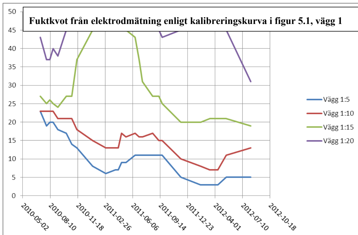
FIG 6.5. Kalibrerad fuktkvot på olika djup i vägg 1.
