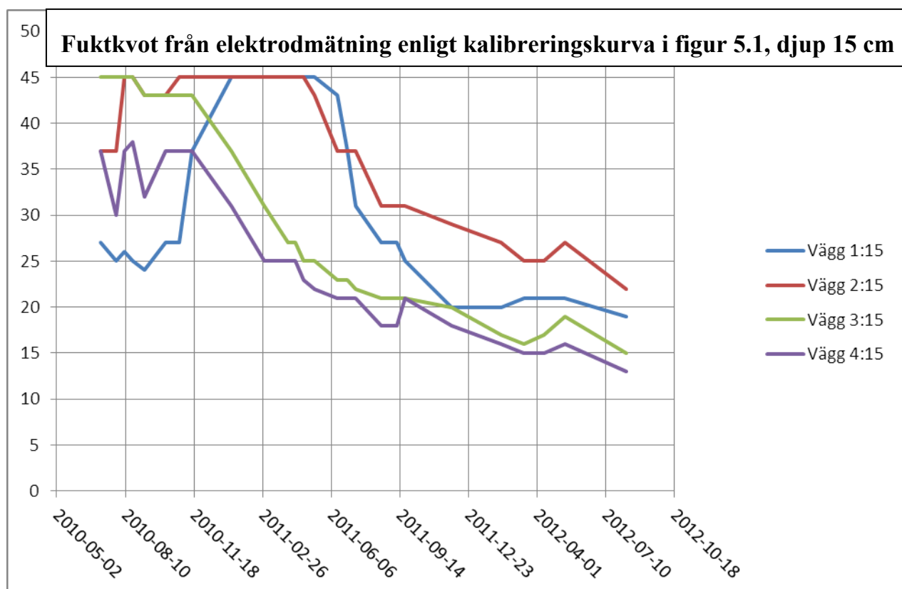
FIG 6.15. Kalibrerad fuktkvot på djupet 150 mm i de olika väggarna.
