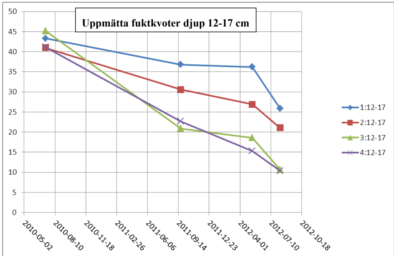
FIG 6.23. Fuktkvot på djupet 120-170 mm i de olika väggarna.
