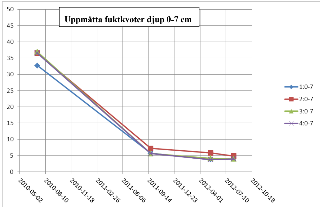
FIG 6.21. Fuktkvot på djupet 0-70 mm i de olika väggarna.
