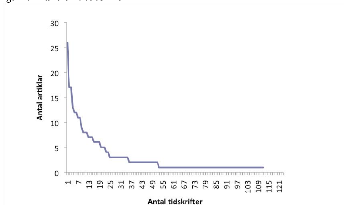
Figur 1. Antal artiklar/tidskrift
