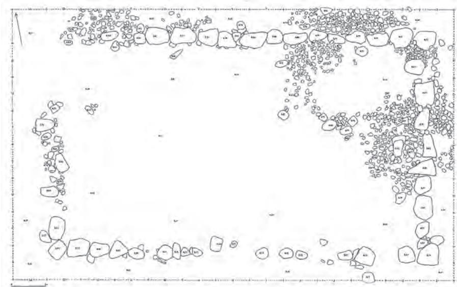
Figur 5.18. Uppmätning av grunden till Pata kapell i samband med undersökningen 1990. Ritning Lars Ersgård. Ur Klackenborg 2001:202.
