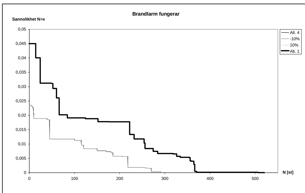
Figur 23. Känslighetsanalys: Sannolikhet att brandlarm fungerar.
