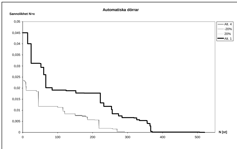
Figur 24. Känslighetsanalys: Sannolikhet att automatiska dörrar fungerar.
