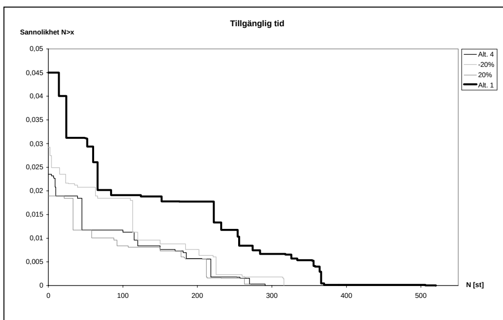
Figur 28. Känslighetsanalys: Tillgänglig tid för evakuering.
