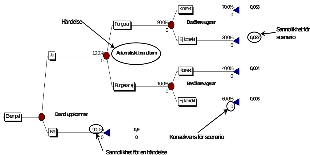
Figur 8. Exempel på händelsetråd.
