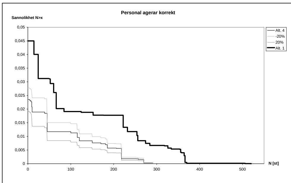
Figur 25. Känslighetsanalys: Sannolikhet för att personal agerar korrekt.
