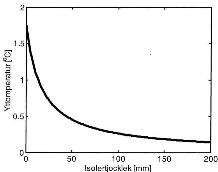
Figur 7.1: Ytemperatur som funktion av isolertjocklek. Vid mindre isolertjocklekar varierar yttemperaturen kraftigt jämfört med större tjocklekar.
