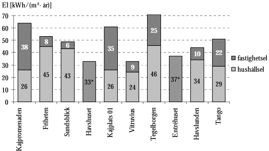
Figur 5:9 Uppmått hushållsel och fastighetsel för de tio fastigheterna. Värden för Havshuset och Entréhuset inkluderar både hushållsel och fastighetsel.
