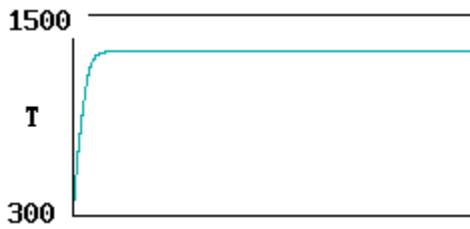
Figur E.4, Temperaturkurva (K) från simulering av heptanförsök 3 med Flashover A1. Diagrammets hela längd motsvarar 120 sekunder. Observera den mycket snabba temperaturstegringen i försökets början /E.1/.
