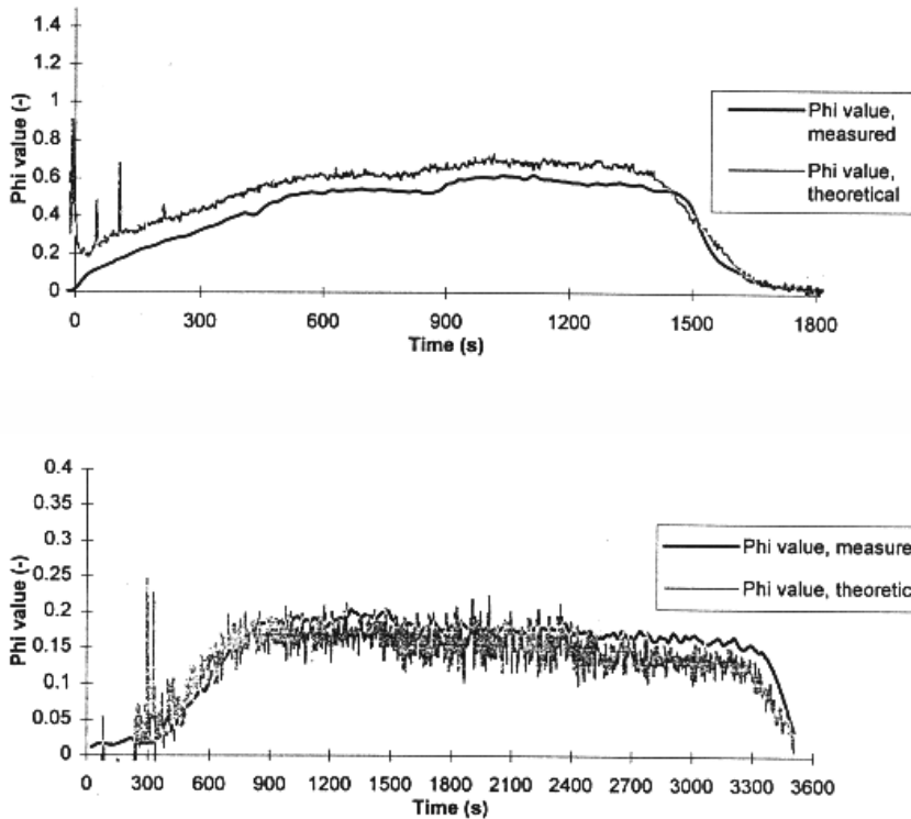
Figur C.5, och C.6, Jämförelse av \Phi -värden, uppmätta med speciell \Phi -mätare respektive beräknade /C.2/.
