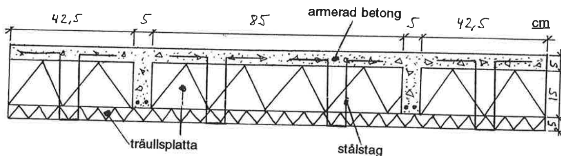
Figur 3. Tak med bärande stomme av betong och värmeisolering av träullsplattor. Köldbryggorna bryts av genom ett heltäckande undre skikt av träullsplattor.
