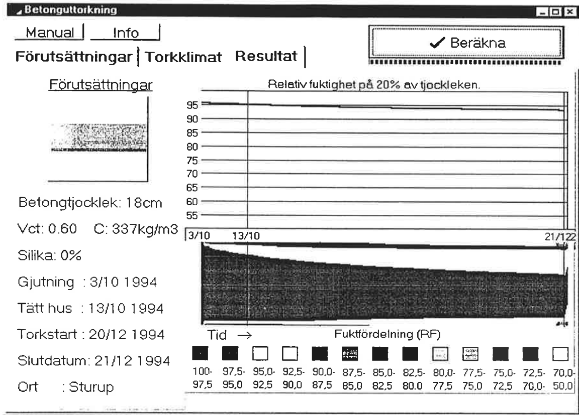
Studie 6 - Uttorkningsförlopp för betong med vct 0,60 (lab. vct 0,60)
