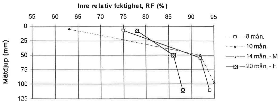
Figur 22 - Fuktprofiler för vattenhärdad, rå betong, vct = 0.69. E = emissionsmätning; M = mattlinning.
