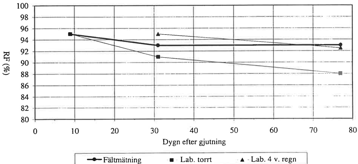
Studie 6 - Uttorkningsförlopp för betong med vct 0,60 (lab. vct 0,60)
