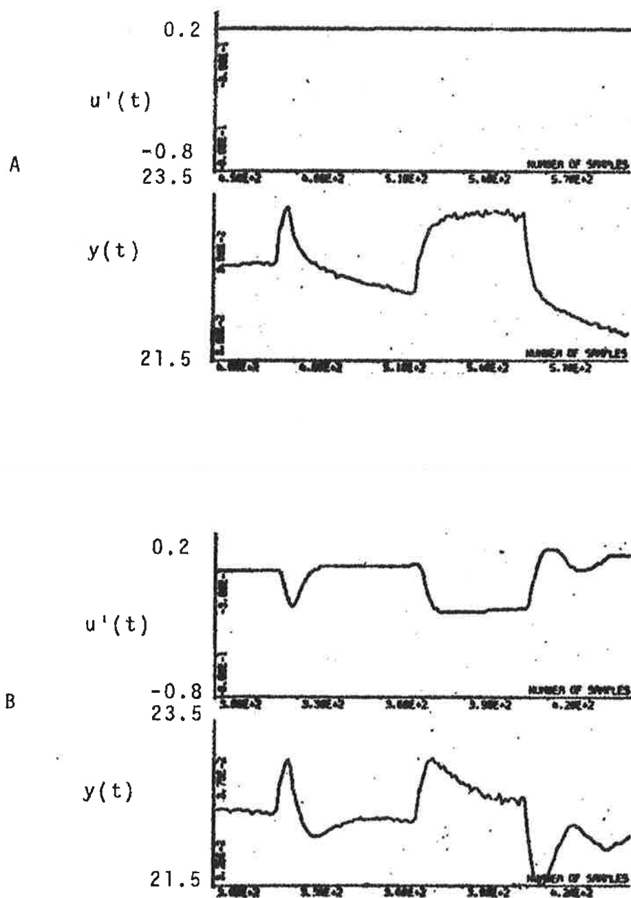
Figur 8.3.5. Experiment utan någon reglering A och med analog PI-regulator B. Störeffekten är på 4 kW. Försökslängden per regulator är 150 minuter. u'(t) betecknar ventilens läge i volt (-0.9 volt helt stängd och 0.9 volt helt öppen). y(t) betecknar rumslufttemperaturen i ^{\circ}\text{C} . Börsvärdet är 22.5^{\circ}\text{C} .
