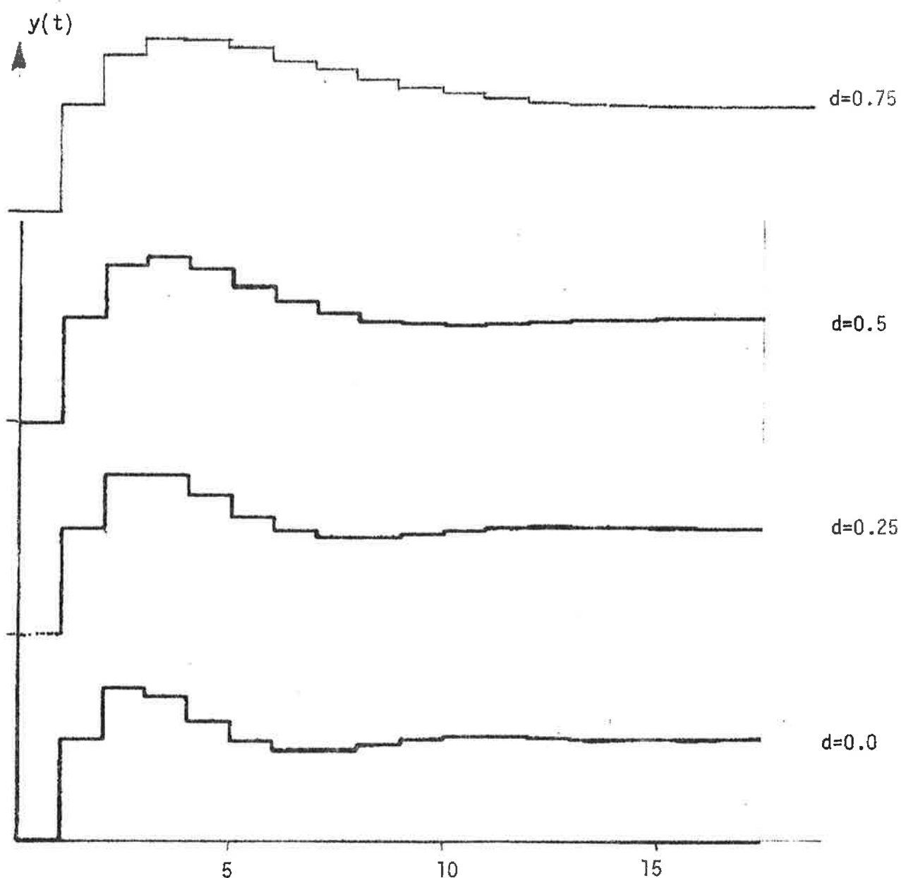
Figur 6.6.2 Exempel på dämpning av kvotregulatorn. Processen, som regleras, har pulsöverföringsfunktionen H(z)=(1-a)/(z-a) . Insignalen u(t) är begränsad till intervallet (0,1) . Det slutna systemets utsignal y(t) har ritats upp förskjuten med en enhet mellan varje exempel. Börvärdet är 0.5. Regulatorn är följande
