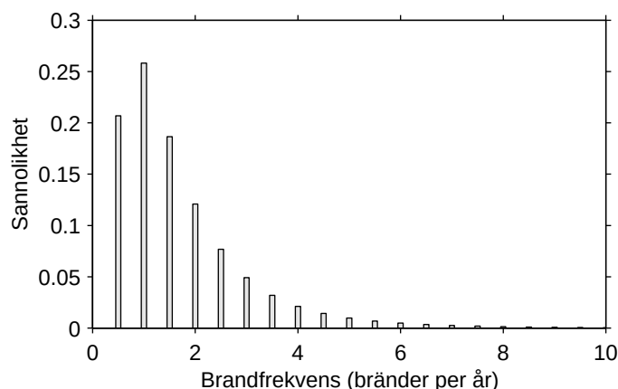
Figur 3 Exempel på apriori-fördelning för brandfrekvensen.
