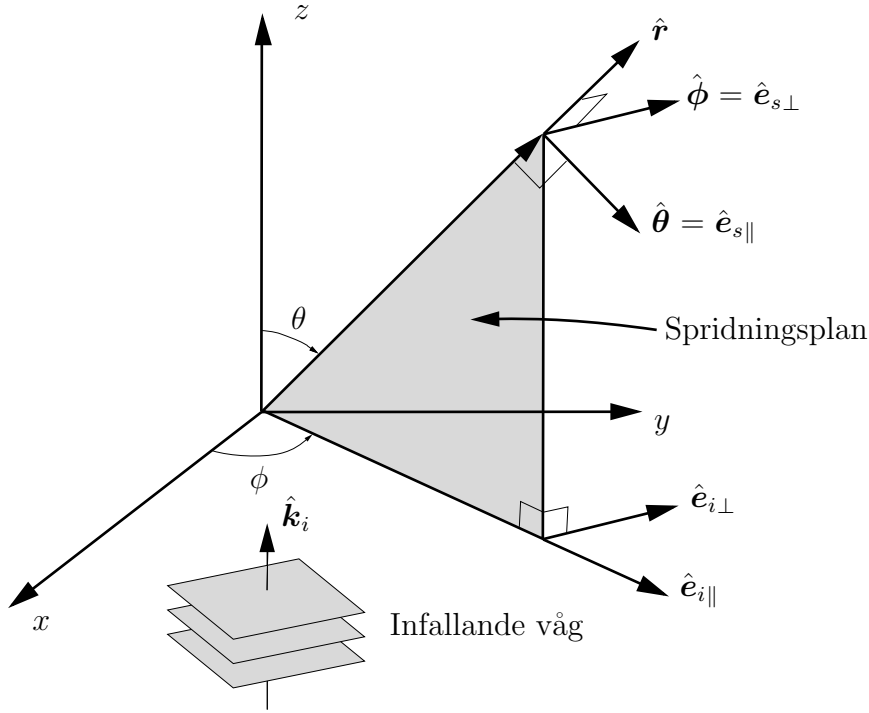
Figur 3.4: Definition av spridningsriktningar. I figuren är den infallande vågens utbredningsriktning vald till \hat{z} , vilket leder till att \hat{e}_{i\perp} = \hat{e}_{s\perp} = \hat{\phi} , \hat{e}_{s\parallel} = \hat{\theta} och \hat{e}_{i\parallel} = \hat{\rho} .
