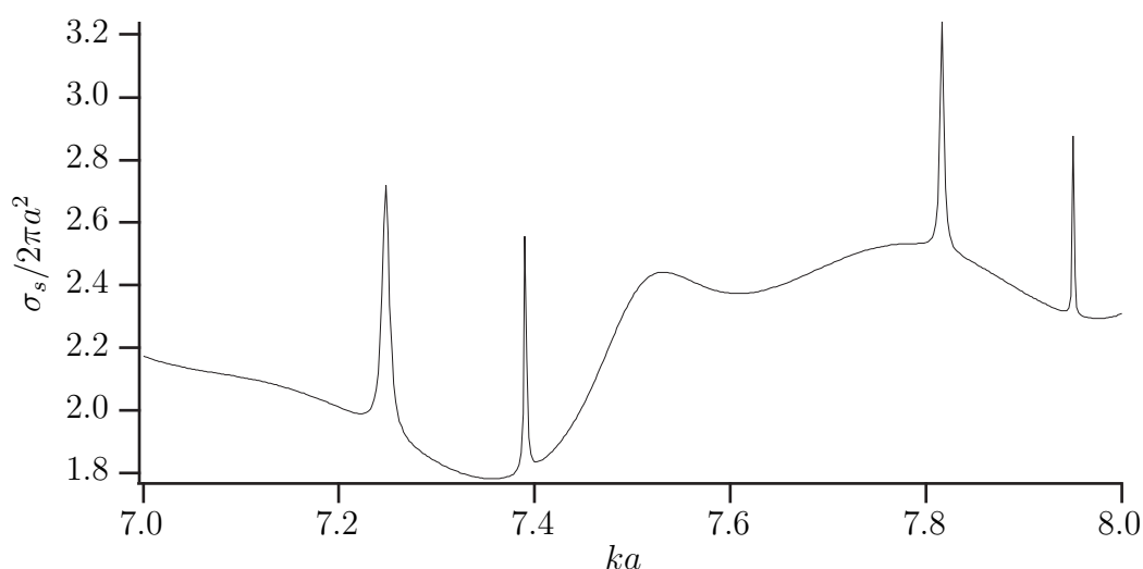
Figur 3.27: Det totala spridningstvärnsnittet \sigma_s/\pi a^2 för en dielektrisk sfär. Sfärens materialparametrar är \epsilon = 4 och \mu = 1 (relativa värden jämfört med omgivande material). Notera normeringen.
