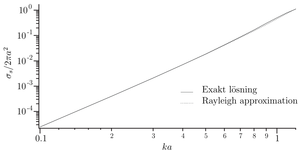
Figur 3.23: Det totala spridningstvärnsnittet \sigma_s/2\pi a^2 för en cirkulär skiva med radie a i långvågsgränsen. Den infallande planvågen infaller vinkelrätt mot diskens plan. Notera log-log skalan och normeringen.
