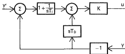
Fig. 3.1. Blockschema för en PID regulator. Regulatorn har två in-signal, mätsignalen y och referensvärdet y^r . Regulatorns utsignal u är processens styrsignal.
