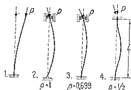
Fig :32a. Knäckning vid ändrad krafteriktning under deformationen
