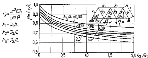
Fig :55v. [118]. Rambärverk i form av fem liksidiga triangelväld
