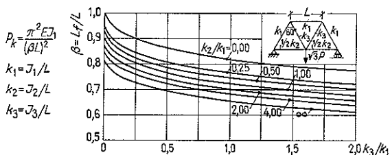
Fig :55u. [118]. Rambärverk i form av tre liksidiga triangelväld
