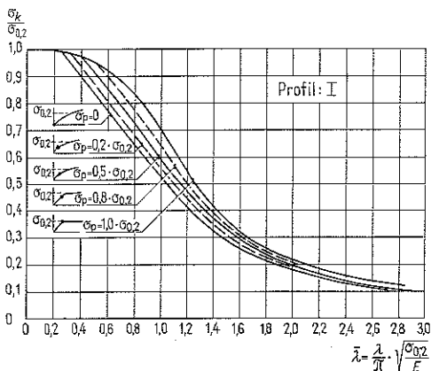
Fig :34d. Knäckningskurvor vid varierende förhållande \sigma_p/\sigma_{0,2} för sträva med ideellt I-tvårsnitt och av material med krökt \sigma - \epsilon -kurva av för aluminiumlegeringar representativ typ. Knäckning i styva riktningen. Initialexcentricitet enligt Dutheil [20]
