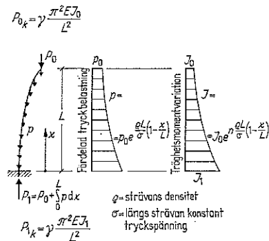
Fig :354d. Egenviktsknäckning av sträva med sektionsutformning som svarar mot i hela strävan konstant tryckspänning. [43]
