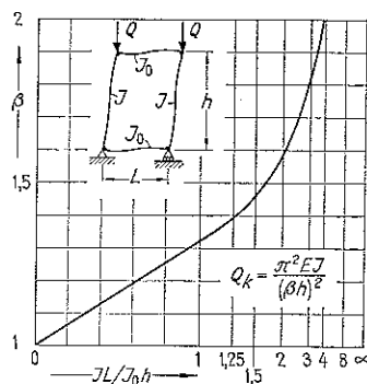
Fig :55s, t.h. [32]. Sluten ram
