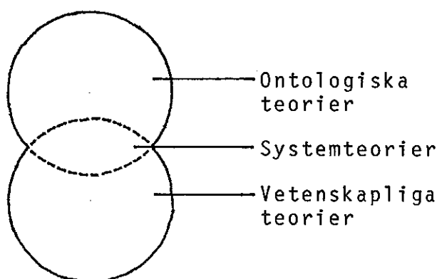
Figur 1.4. Relationen ontologi-systemteori-vetenskap.
