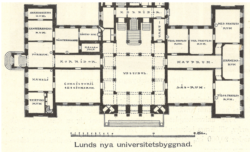
Planritning över östra delen av 1882 års universitetshus med universitetsledningens och förvaltningens lokaler i den södra änden av byggnadens "vardagsaxel". Bildkälla: Lunds universitet 1872–1897 (Lund 1897).
