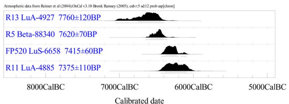
Fig. 15. Kalibrerade ^{14}\text{C} -värden från fyndplatser i detritusgyttjan.
