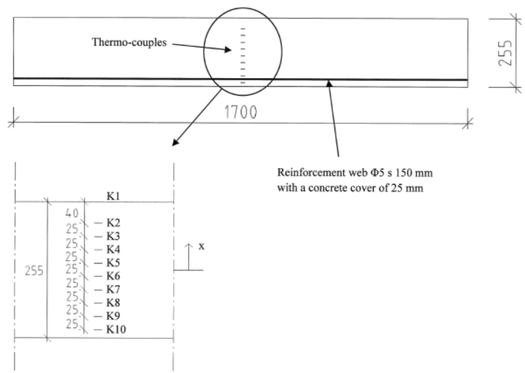
Figur 6.2. Placering av givare i betongplattan (Larsson 2009)
