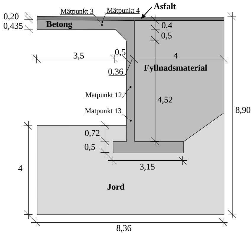
Figur 4.2. Strukturmodell över brotsvärsnitt och intilliggande jord och fyllnadsmaterial, som använts i simuleringar.
