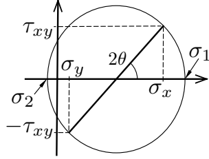
Figur 11: Mohrs cirkel för analys av spänningar. a) visar det fysiska planet b) visar ett plan för normalspänning \sigma resp. skjuvspänning \tau . Vinkeln är \theta mellan x - y riktningarna och 1-2 riktningarna i det fysiska planet.
