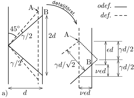
Figur 15: a) Töjning och skjuvning vid enaxlig dragning. Den ursprungligen rätvinkliga triangelns spetsiga hörn är 45^\circ (heldragen). b) betraktelse av den i a) inringade delen
