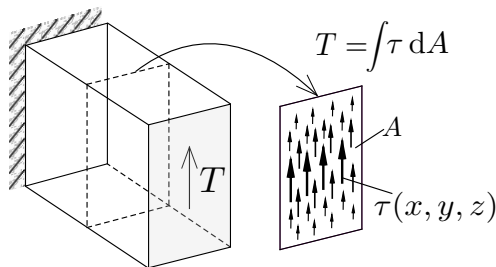
Figur 6: Ett prisma belastat av skjuvkraften T erhåller en genomsnittlig skjuvspänning \tau = T/A . Eftersom skjuvspänningen försvinner på de fria över- och underytorna blir spänningen aldrig homogent fördelad som i fallet med enaxlig dragbelastning.
