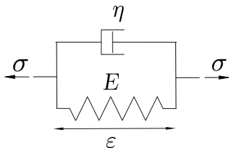
Figur 17: Kelvin-Voigt material
