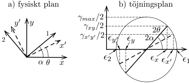
Figur 4: Mohrs cirkel. a) visar det fysiska planet b) visar ett töjningsplan med axlar för töjning \epsilon resp. skjuvning \frac{1}{2}\gamma . Vinkeln är \theta till ett godtyckligt roterat koordinatsystem x' - y' (ekv. 13, 14 och 17) och \alpha är vinkeln till huvudtöjningsriktningarna 1-2, ekv. 19. Notera att vinklarna är dubbelt så stora och motriktade i Mohrs cirkel.
