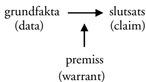
Figur 2 Toulmins argumentationsmodell
