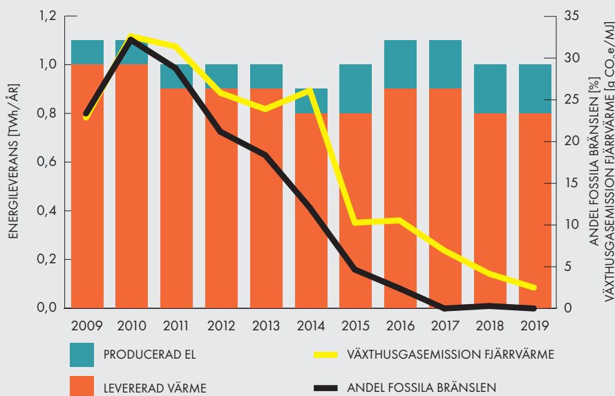
FIGUR 2. ENERGILEVERANS, ANDEL FOSSILA BRÄNSLEN OCH KLIMATPRESTANDA I KRAFRINGEN ENERGIS FJÄRRVÄRMENÄT 2009-2019
